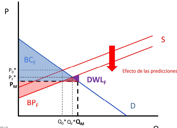
Modelo teórico del cambio en la curva agregada de oferta en el sector eléctrico por la existencia de información meteorológica. Estudio del Sector Infomediario 2014. Parte III.
